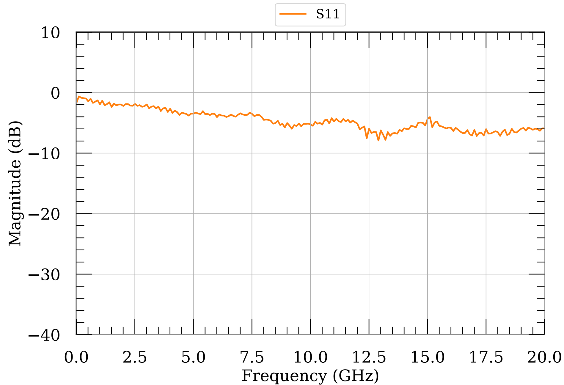
LNA S-params module012
